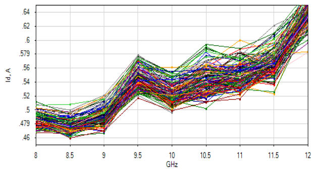
Ток потребления (при компрессии на 1 дБ)
