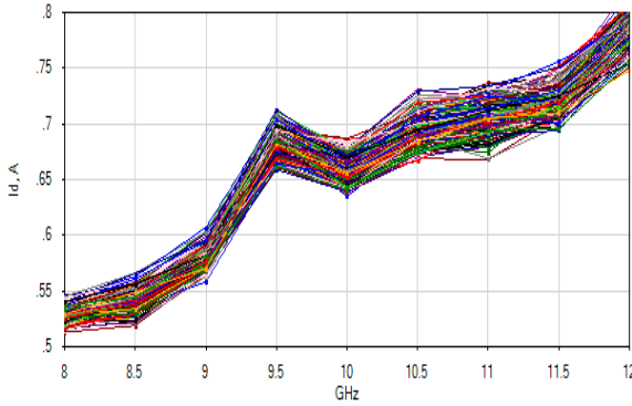
Ток потребления (при компрессии на 3 дБ)
