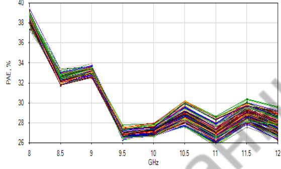
КПД по добавленной мощности (при компрессии на 3 дБ)
