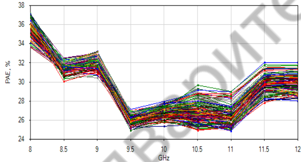
КПД по добавленной мощности (при компрессии на 1 дБ)
